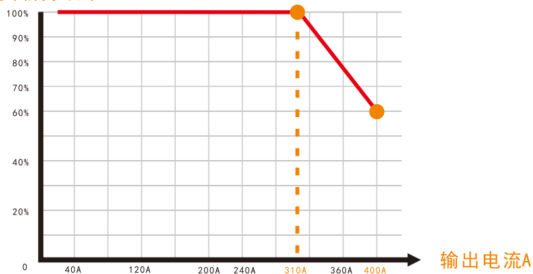
负载持续率 (40°C)
