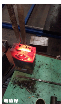
电渣焊
