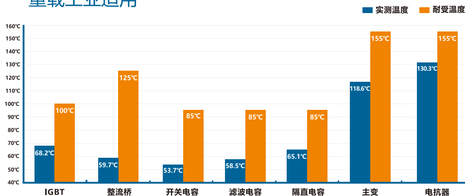
▲ 环境温度40℃，输出1250A/44V，稳定工作4小时，部分关键元器件实测温度数据
